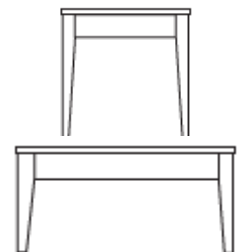
End Table 23"W x 27"D x 23"H Cocktail Table 34"W x 20"D x 16"H
